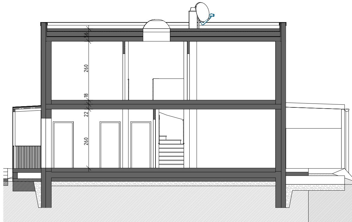
SCHNITT A M1:100
