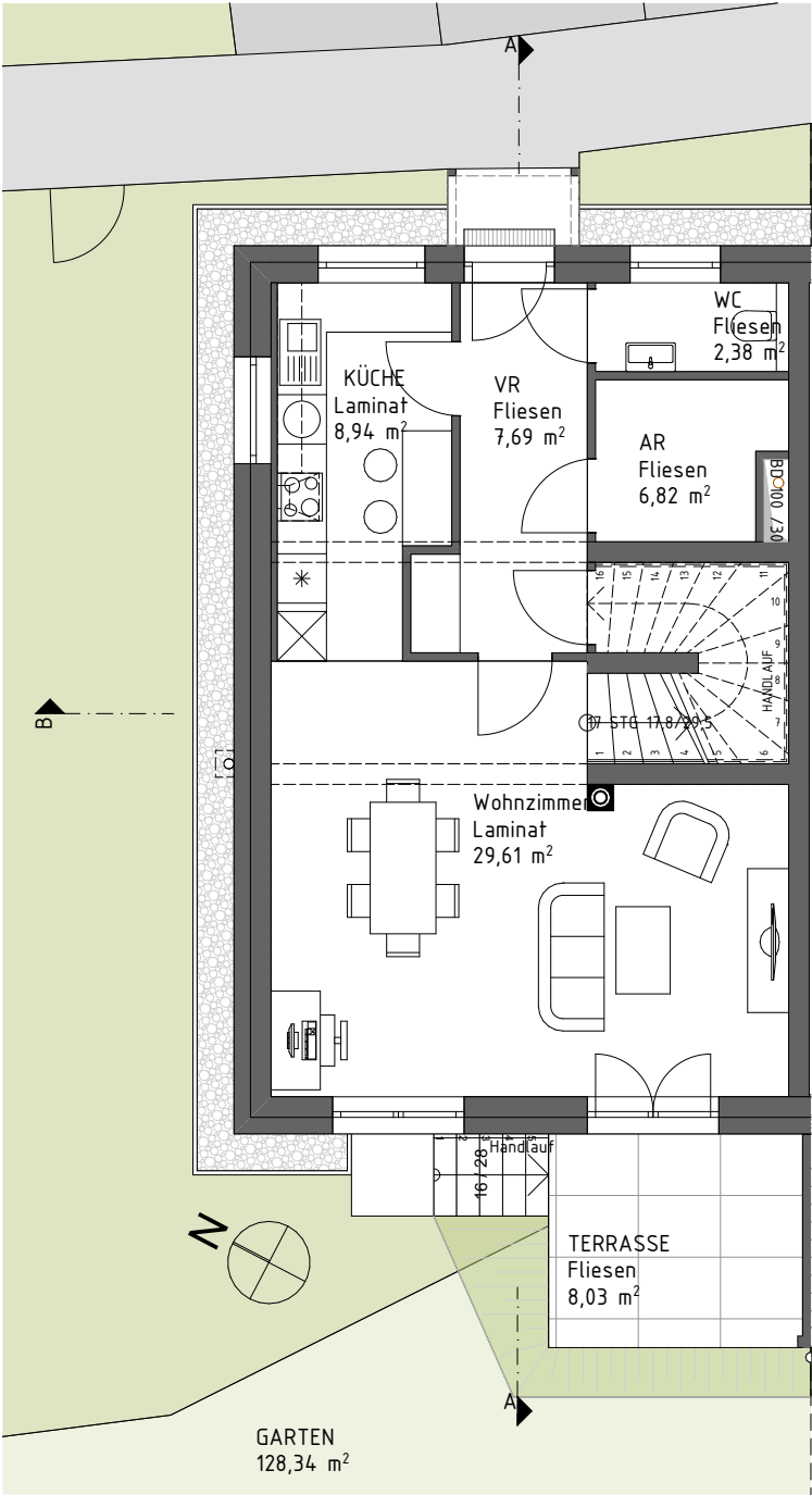
ERDGESCHOSS M1:100
