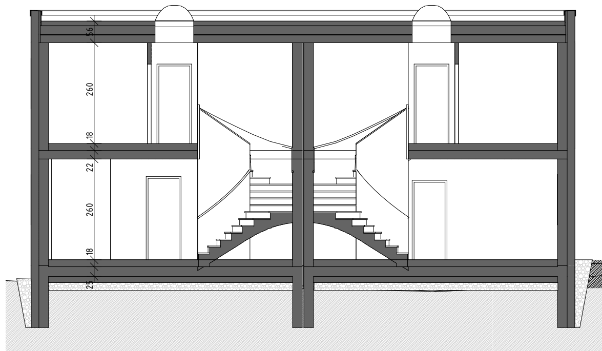
SCHNITT B M1:100
